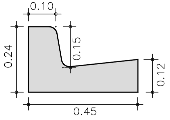
GUIA EXTRUSADA CONCRETO: 0.063 m 3 /m S/ESCALA
