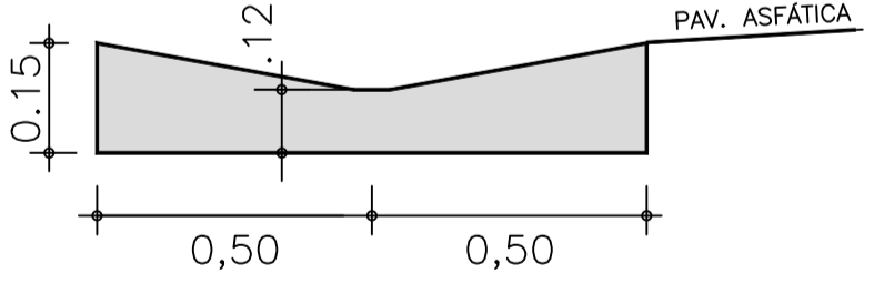
SARJETÃO CONCRETO: 0.182 m 3 /m S/ESCALA
