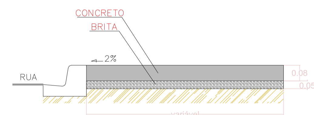
PERFIL - CALÇADA Sem Escala
